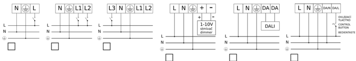
Principiální schéma k připojení a stmívání svítidel / Schematic diagram for connection and dimming of luminaires / Schematischer Schaltplan zum Anschließen und Dimmen von Leuchten
